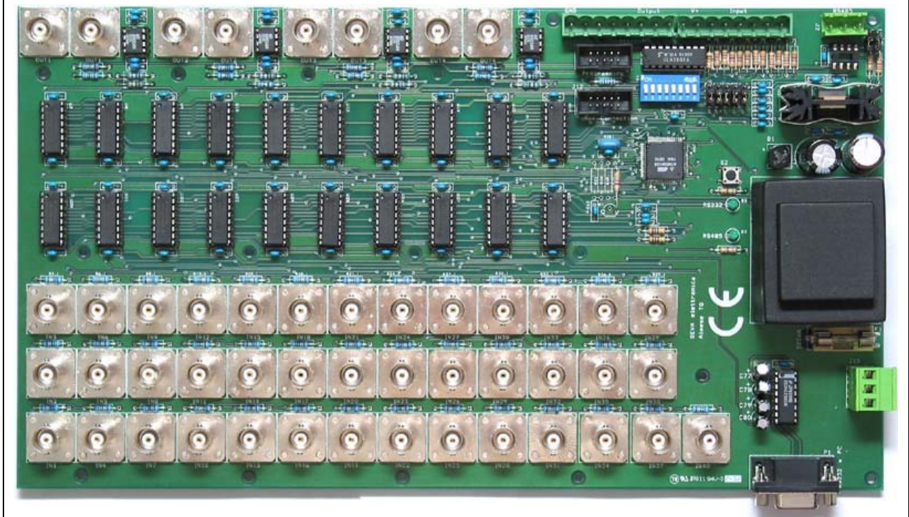
Scheda di switch video, interfaccia joystick e IO, rete485.
